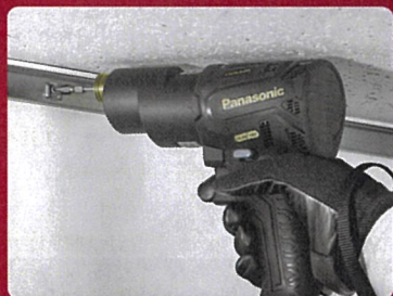
壁際のメタルモールの取り付け
